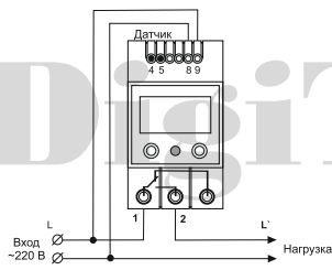
Схема подключения
