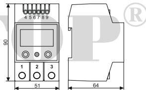
Габаритные размеры
