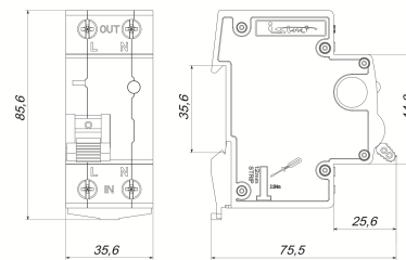
Рис. 3. Размеры УЗДП
